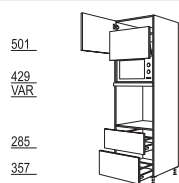
GLO2A-3X
