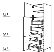
HI*-3X 40/50/60 cm
