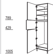
G123G-3X
