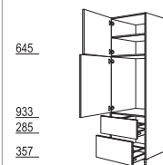
G88A-3X
