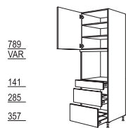
GOS2A-3X
